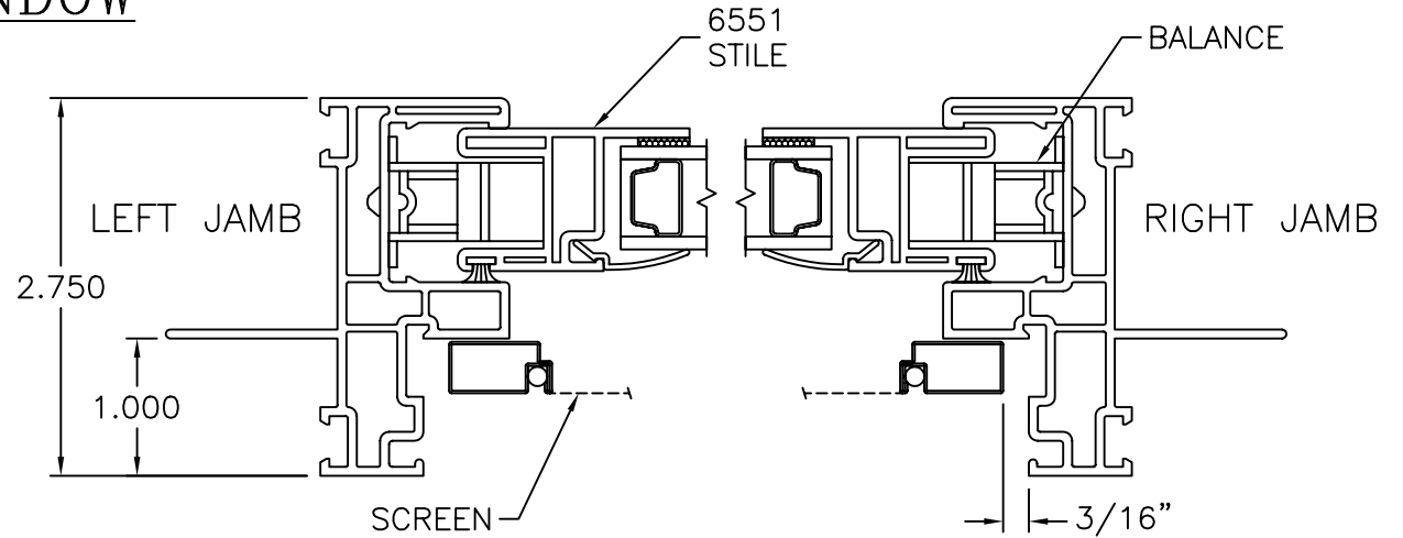
HORIZONTAL SECTION (VENT - LITE)
